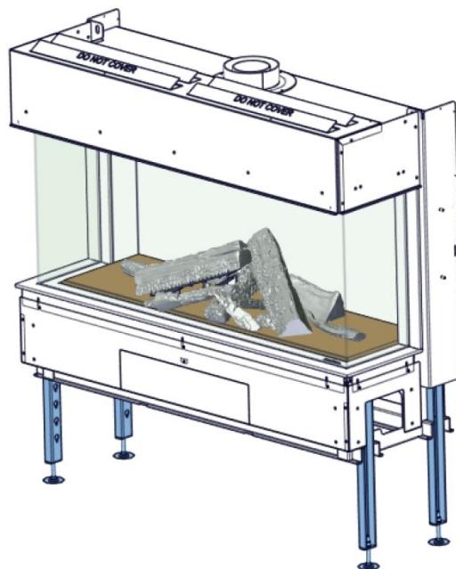
Abb. 5: Ausrichtung mittels höhenverstellbarer Füße
