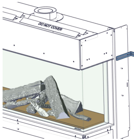
Abb. 6: Befestigung an der Rückwand
