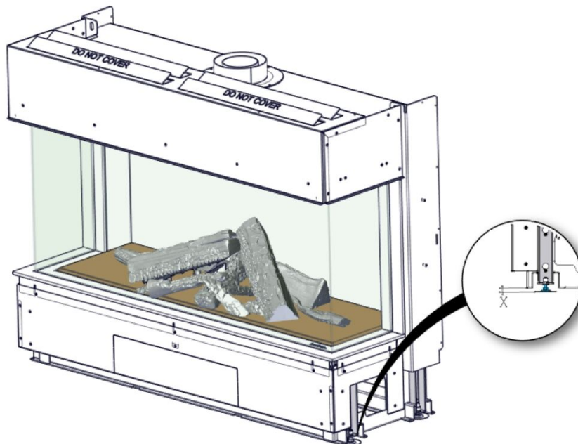
Abb. 4: Ausrichtung mittels Stellfüßen
