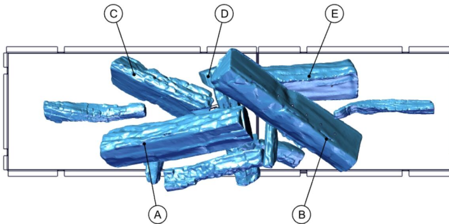
Abb. 10: Positionen der Holzimitate und Brennerleisten
